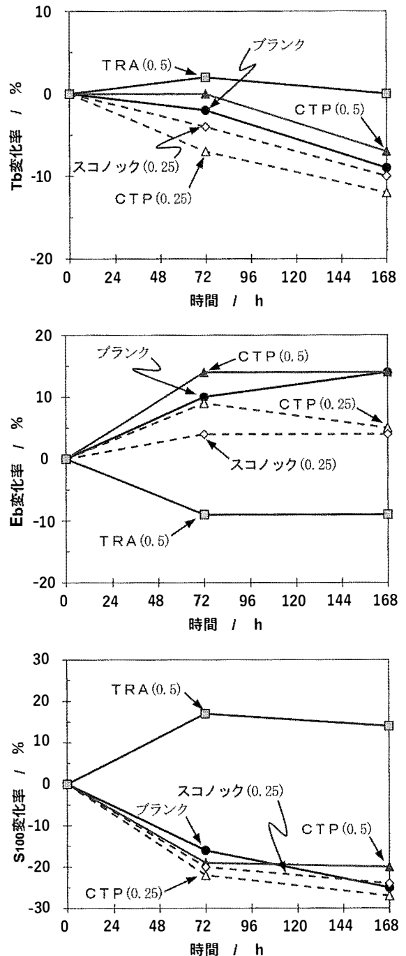
図1 熱老化時間と加硫ゴム物性の変化率
