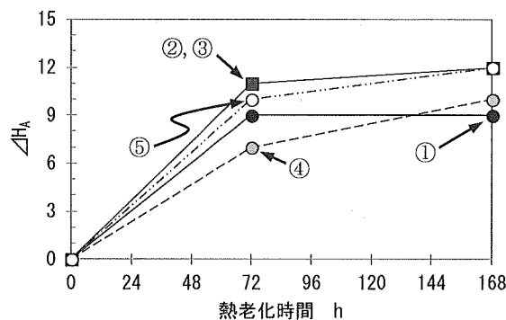
図3 熱老化後の H_A の変化
