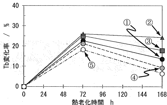
図1 熱老化後のTb変化率
