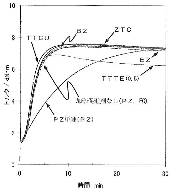
図1 加硫曲線
