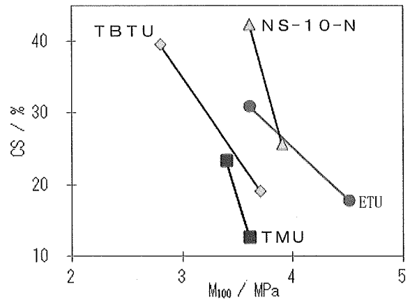
図1 圧縮永久ひずみ(120℃×72時間)とM 100 の関係
