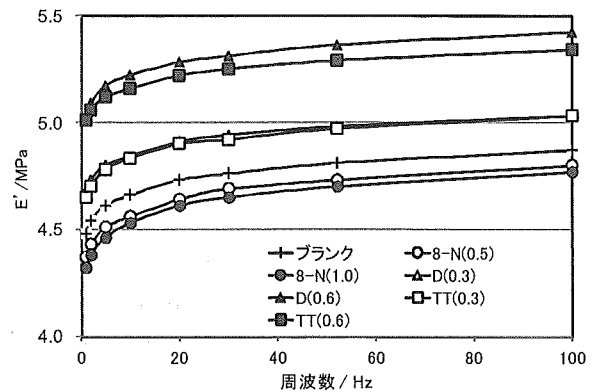
図2 動的弾性率 ( E' ) の周波数分散
