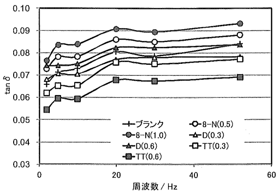
図1 \tan \delta の周波数分散
