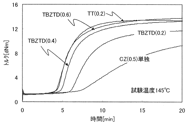
図2 CZ/TBZTD(変量)併用の加硫曲線図
