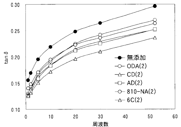
図4 老化防止剤配合加硫ゴムの損失係数( \tan \delta ): 120°C x 70時間熱老化後
