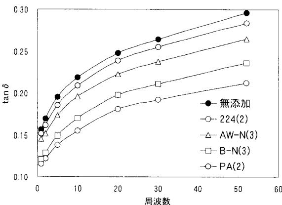
図3 老化防止剤配合加硫ゴムの損失係数( \tan \delta ): 120°C x 70時間熱老化後
