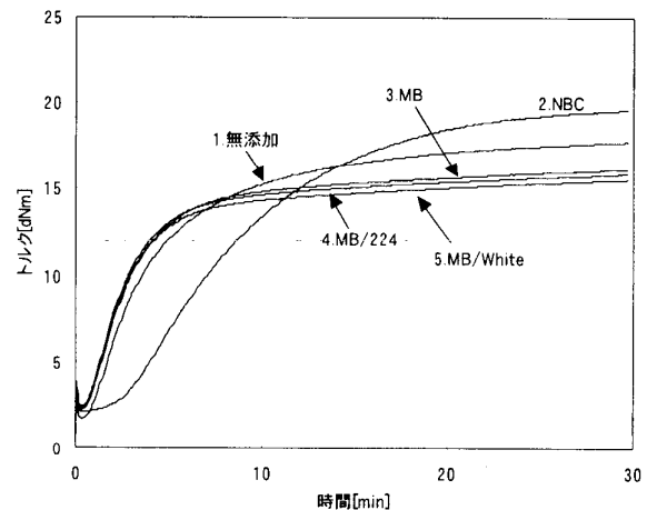
図1 MDR加硫曲線図-1
