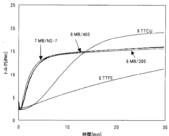
図2 MDR加硫曲線図-2
