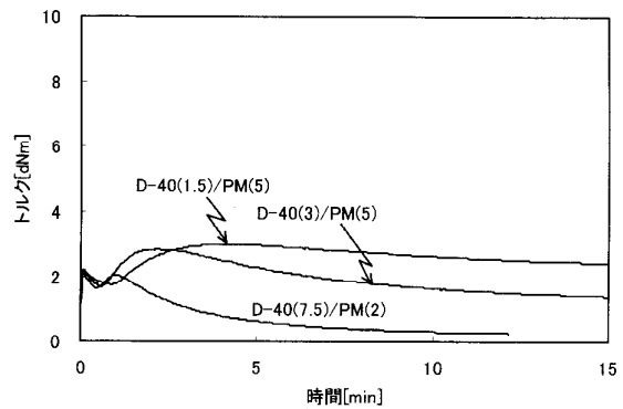
図1 ブチルゴムの過酸化化物加硫に対するPMの効果
