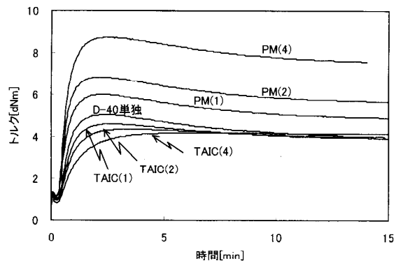
図3 部分架橋ブチルゴムの過酸化化物加硫に対するPMの効果 (D-40; 3phr)
