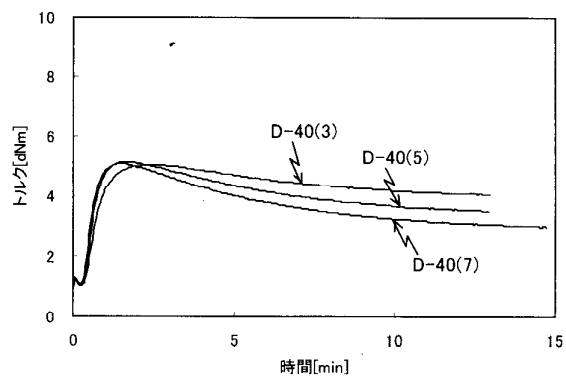
図2 部分架橋ブチルゴムの過酸化化物加硫 (D-40変量)
