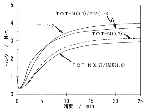
図2 加硫曲線 (TOT-N/架橋助剤の併用)
