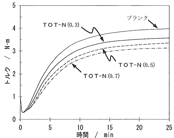
図1 加硫曲線 (TOT-Nのスコーチ防止効果)
